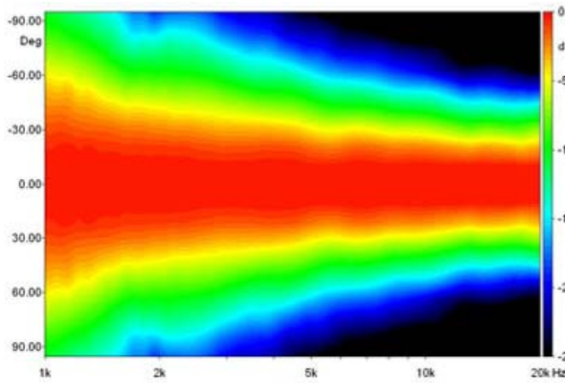
Horizontal Beamwidth
